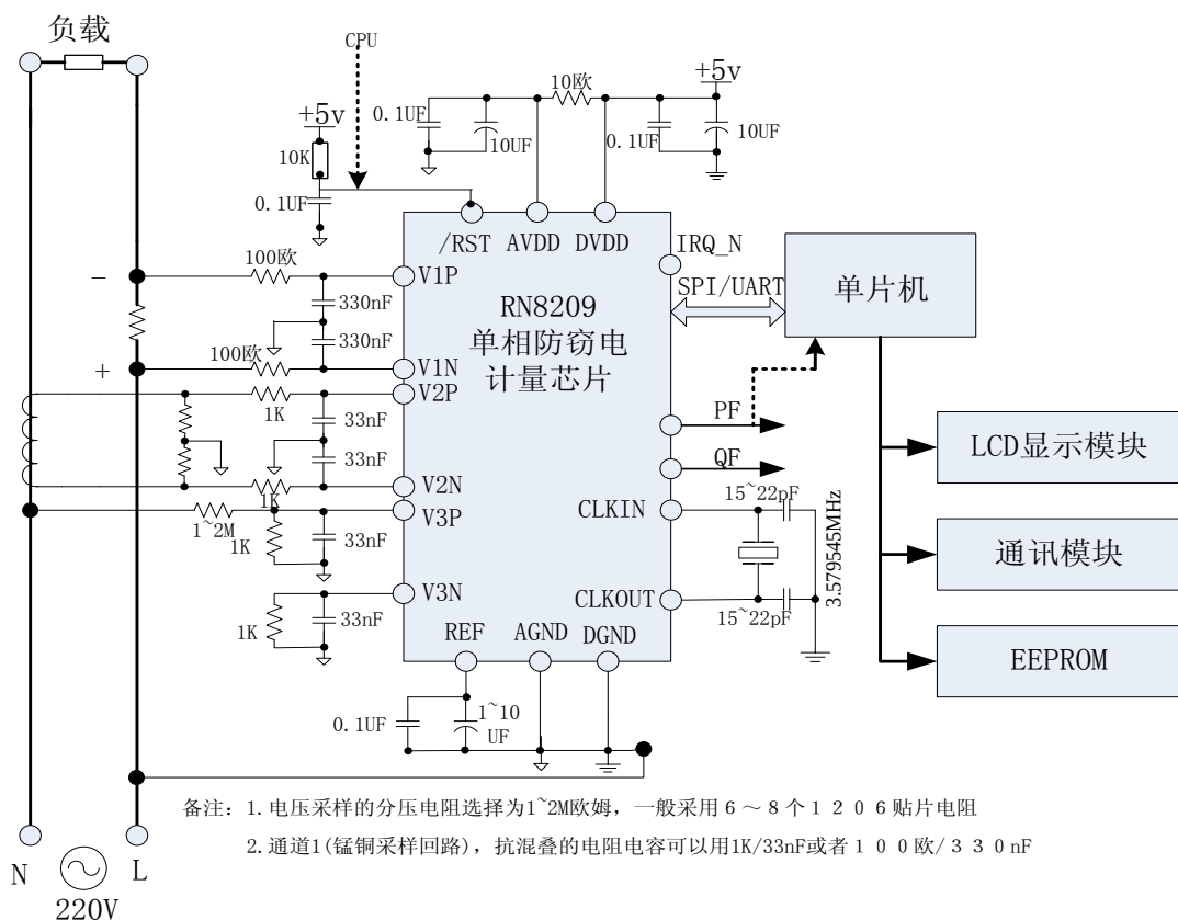
用 RN8209D 设计的单相电能表参考原理框图
