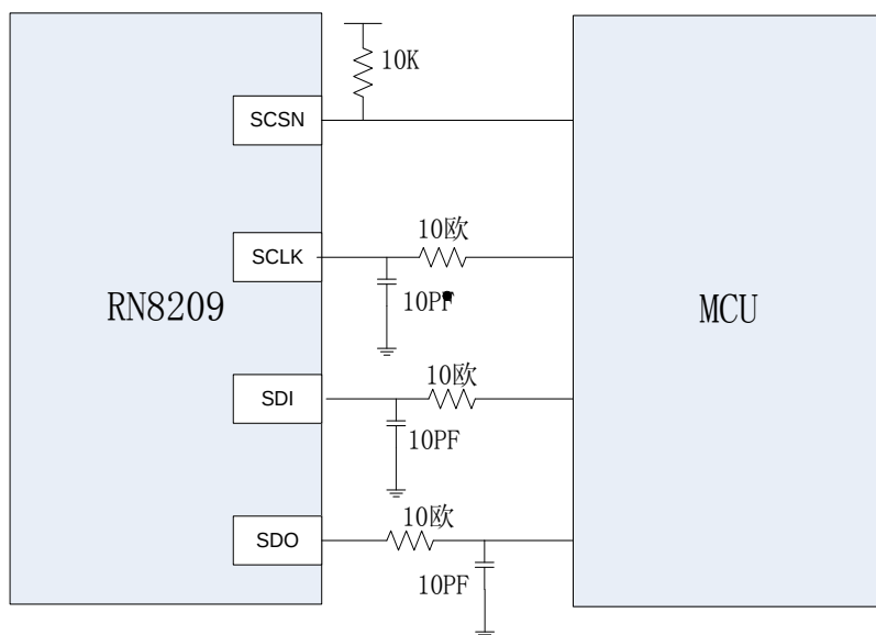
SPI 接口参考电路原理图
