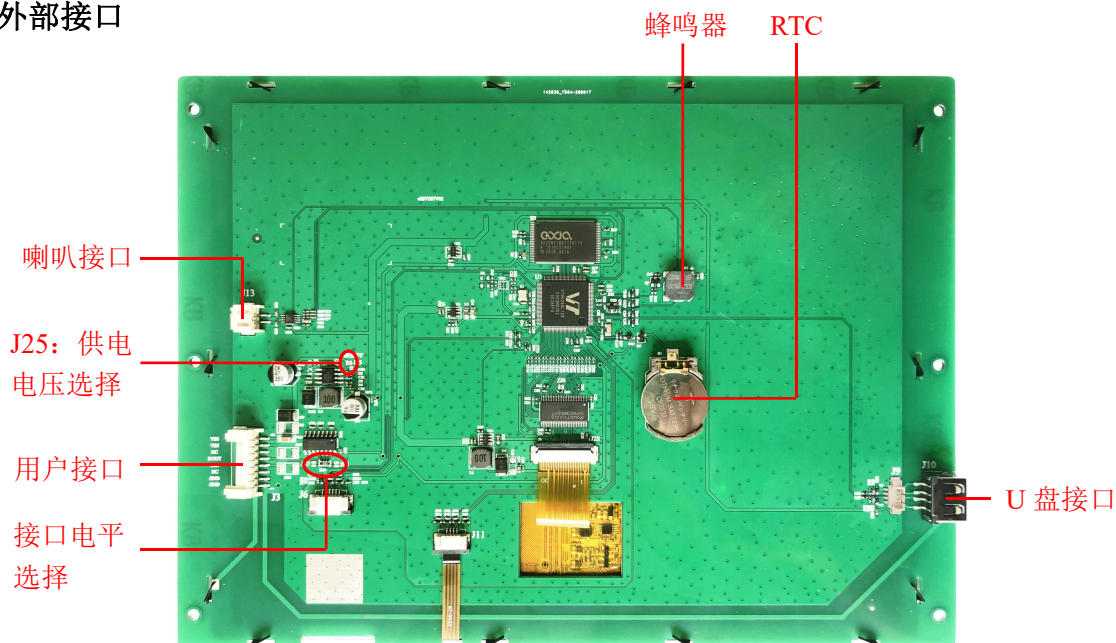
图 1 产品外观及硬件配置图
